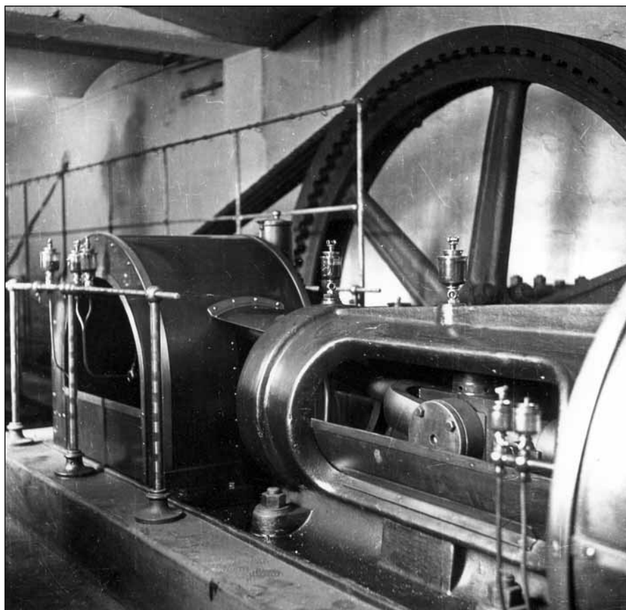
Pohled na klikový mechanismus a lanový setrvačnick rapotínského parního stroje, 1968. (foto Karel Miloš)
