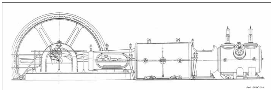
Celkový boční pohled na parní stroj rapotinské sklárny, 1968. (nakreslil Karel Miloš)
